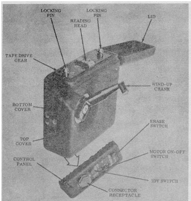
Figure 1-4. KE-8B Keyer
